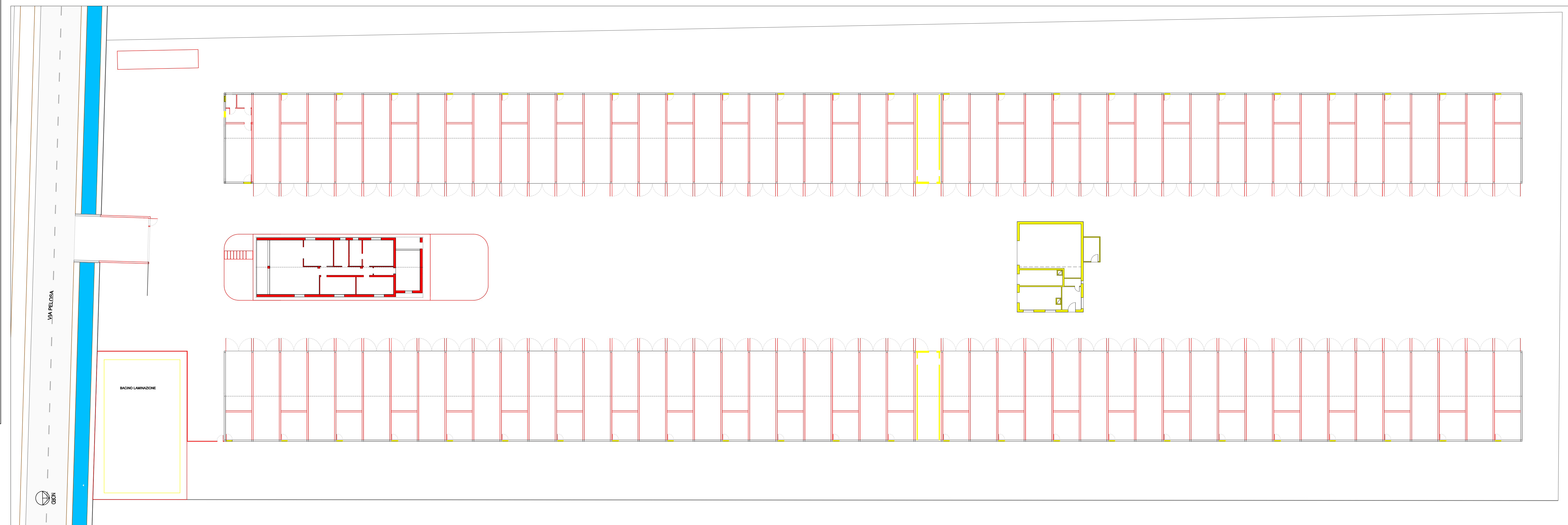
PIANTA DI PROGETTO SCALA 1:200
